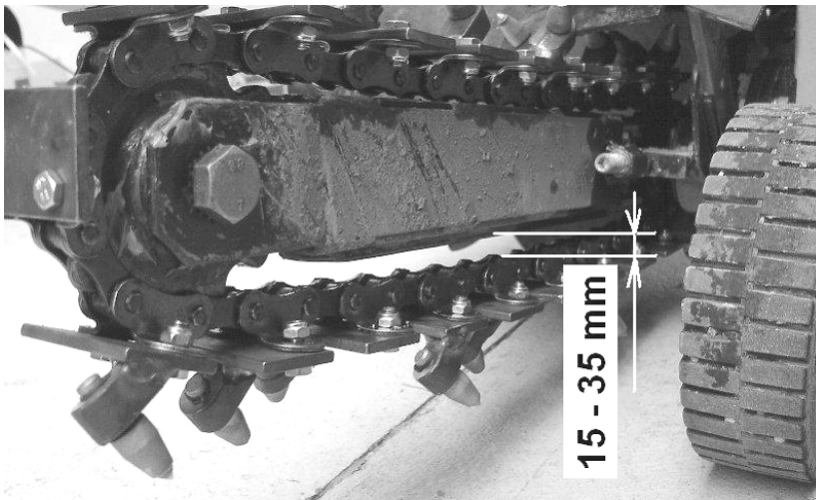
Der empfohlene Kettendurchgang
