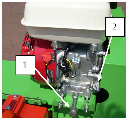
Ablassöffnung (1) und (2) Füllschraube für Motoröl
